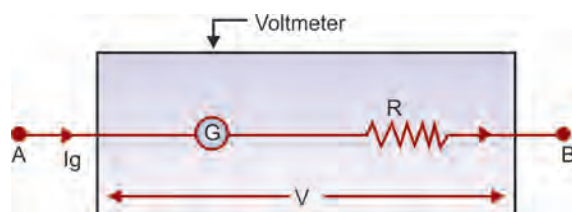
Fig. 1.38: Voltmeter
